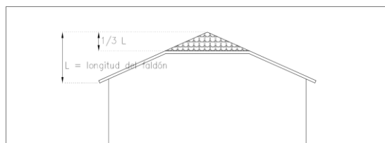
Figura 11: Cubierta tradicional
